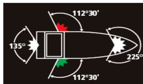
Positionsbeleuchtung für Fahrzeuge mit Maschinenantrieb
